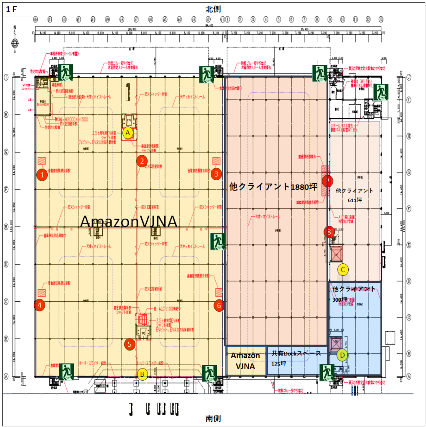
センター構内図面
