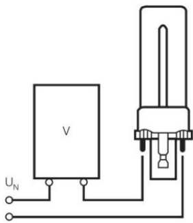
EINZELLEUCHE MIT VORGERÄT
