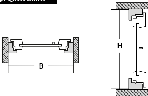
Bsp. Querschnitt
