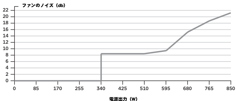
CORSAIR RM850x 内蔵電源ファンのノイズ曲線
