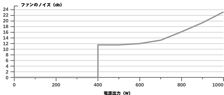
CORSAIR RM1000x 内蔵電源ファンのノイズ曲線
