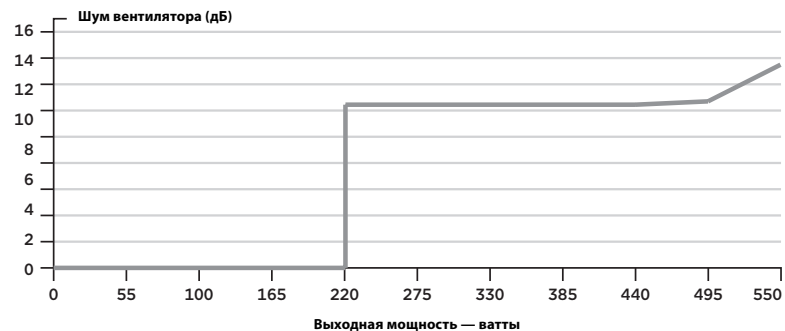
Кривая уровня шума вентилятора блока питания CORSAIR RM550x
