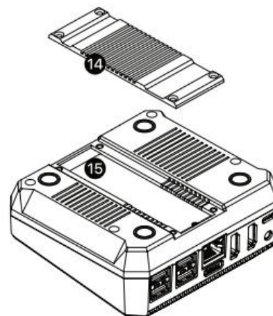
ARGON ONE V3 M.2 NVMe PCIE
