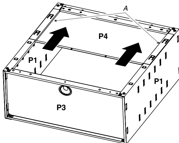
A. Orificios para instalar el soporte de montaje
