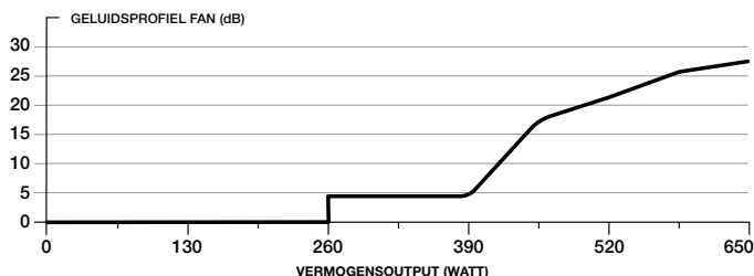
RUISCURVE VAN DE CORSAIR RM650x-VOEDINGSFAN
