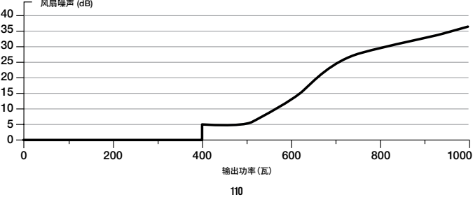
CORSAIR RM1000x 电源风扇噪音曲线
