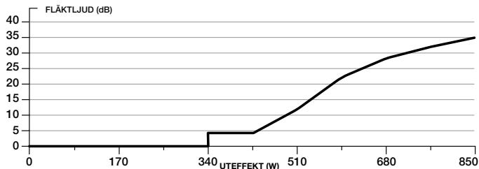
CORSAIR RM850x: BRUSKURVA FÖR NÄTAGGREGATETS FLÄKT
