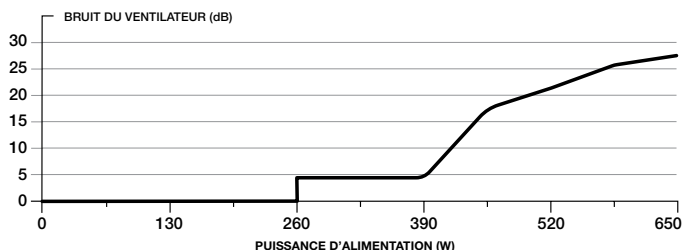
COURBE SONORE DU VENTILATEUR DE L'ALIMENTATION CORSAIR RM650x
