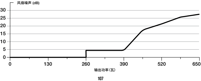
CORSAIR RM650x 电源风扇噪音曲线
