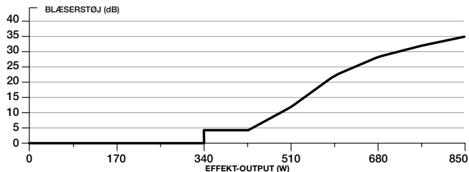
STØJKURVE TIL BLÆSER TIL CORSAIR RM850x-STRØMFORSYNING
