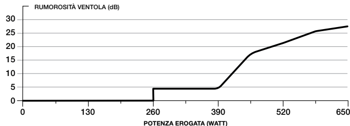
GRAFICO DEL RUMORE DELLA VENTOLA DELL'ALIMENTATORE CORSAIR RM650x
