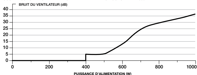
COURBE SONORE DU VENTILATEUR DE L'ALIMENTATION CORSAIR RM1000x
