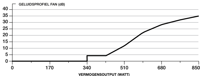
RUISCURVE VAN DE CORSAIR RM850x-VOEDINGSFAN
