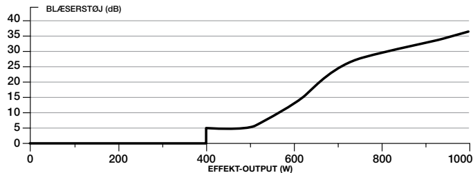
STØJKURVE TIL BLÆSER TIL CORSAIR RM1000x-STRØMFORSYNING
