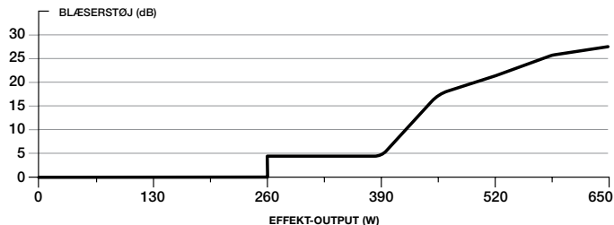
STØJKURVE TIL BLÆSER TIL CORSAIR RM650x-STRØMFORSYNING
