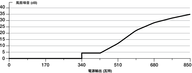
CORSAIR RM850x 電源風扇噪音曲線
