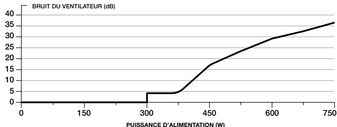
COURBE SONORE DU VENTILATEUR DE L'ALIMENTATION CORSAIR RM750x
