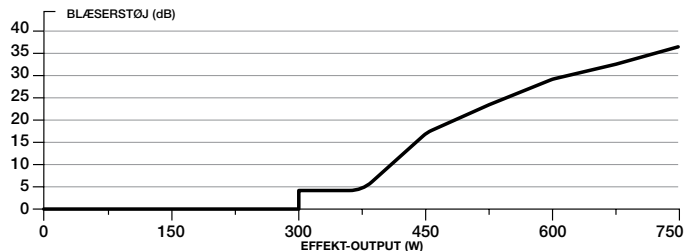
STØJKURVE TIL BLÆSER TIL CORSAIR RM750x-STRØMFORSYNING
