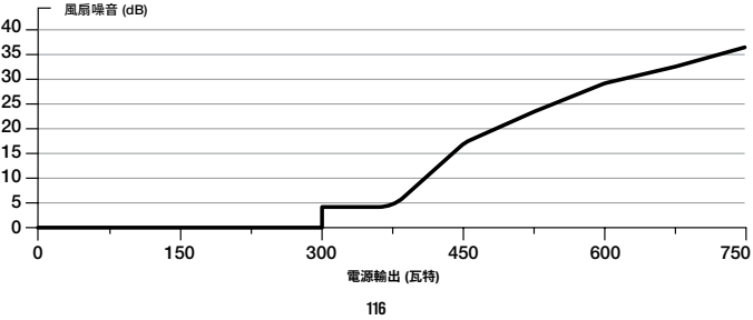
CORSAIR RM750x 電源風扇噪音曲線
