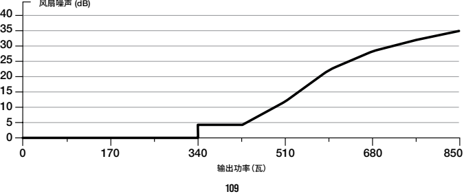
CORSAIR RM850x 电源风扇噪音曲线
