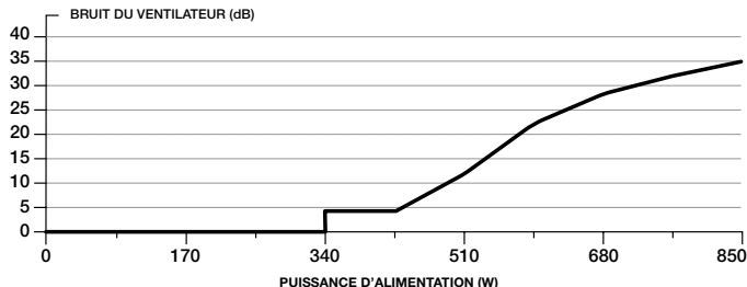
COURBE SONORE DU VENTILATEUR DE L'ALIMENTATION CORSAIR RM850x
