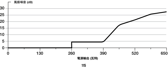
CORSAIR RM650x 電源風扇噪音曲線
