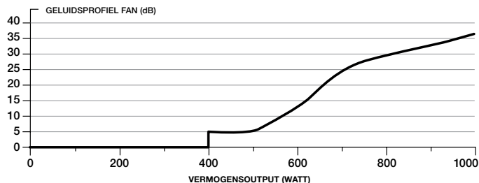
RUISCURVE VAN DE CORSAIR RM1000x-VOEDINGSFAN
