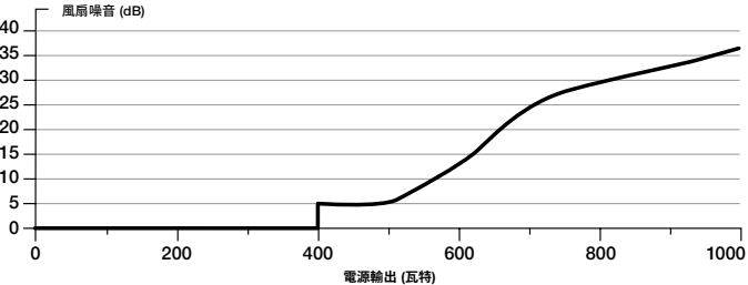
CORSAIR RM1000x 電源風扇噪音曲線
