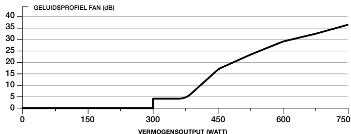
RUISCURVE VAN DE CORSAIR RM750x-VOEDINGSFAN
