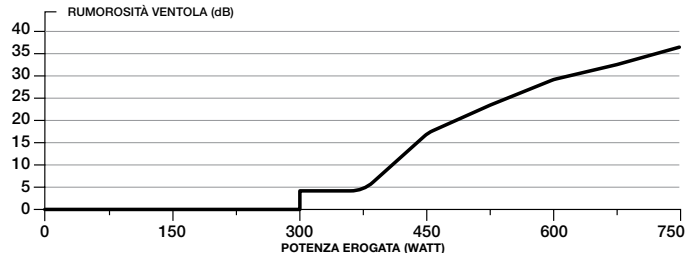
GRAFICO DEL RUMORE DELLA VENTOLA DELL'ALIMENTATORE CORSAIR RM750x
