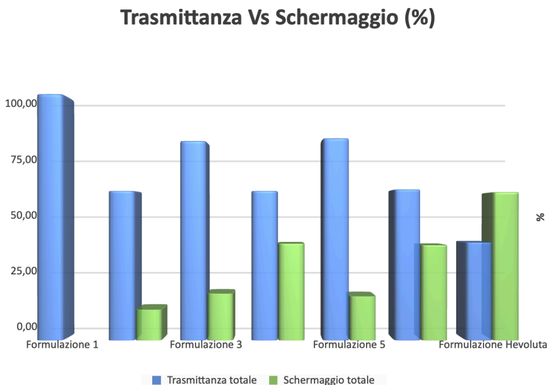
Figura 2: valori di trasmittanza ed assorbimento percentuale della radiazione a confronto.
