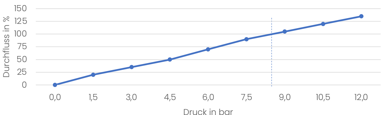
Durchfluss in Abhängigkeit des Drucks an den Membranen
