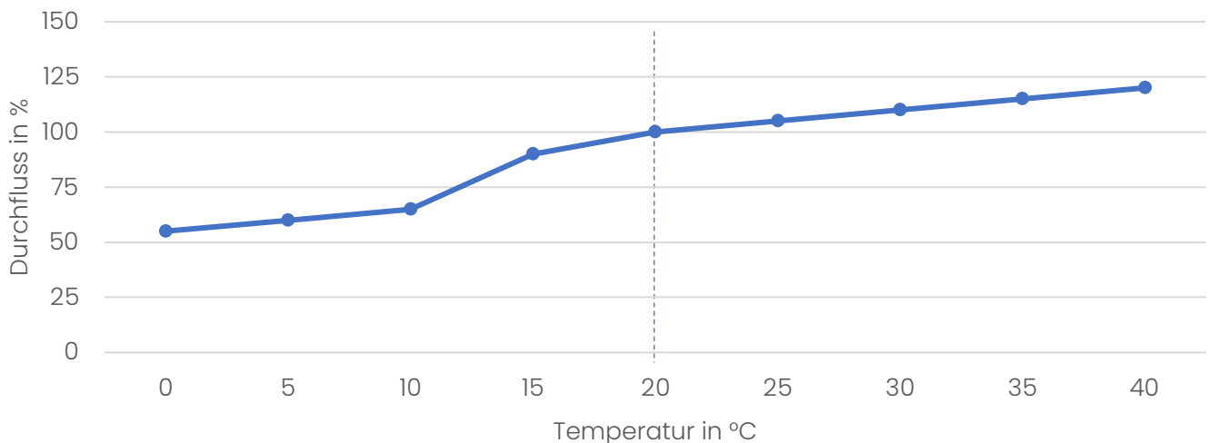
Durchfluss in Abhängigkeit der Temperatur
