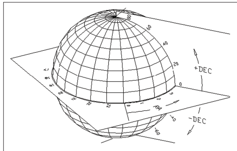
Abb. 14 Die Himmelskugel, von außen betrachtet, mit Angabe von R.A. und DEC.
