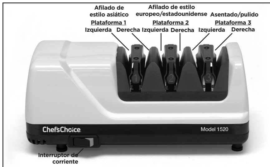
Figura 1. Afiladora Angle Select® - Modelo 1520 de Chef'sChoice® diseñada para afilar cuchillos de estilo asiático, europeo y estadounidense.
