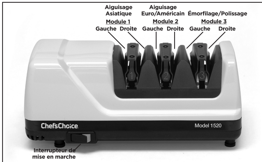
Figure 1. Aiguiser modèle 1520 AngleSelect® Chef'sChoice®, conçu pour aiguiser aussi bien les couteaux de type asiatique que ceux de type euro-américain.
