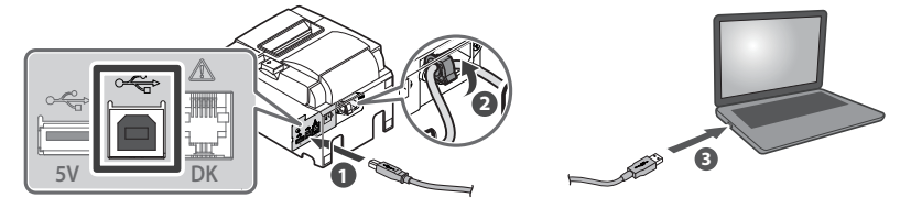
プリンター側プラグ (Type B)
