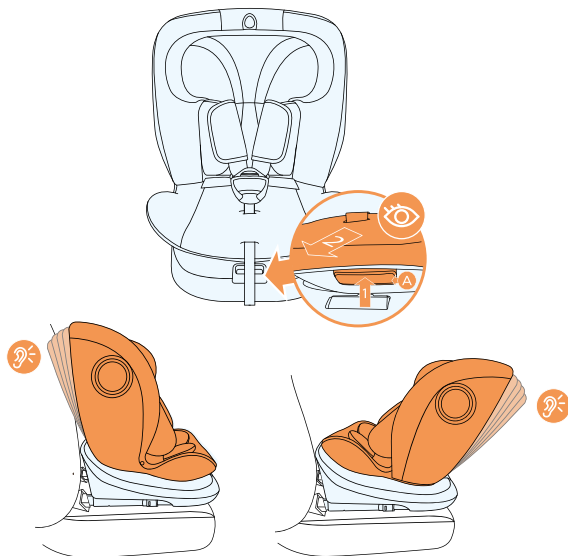
A: Palanca de ajuste del ángulo de inclinación del respaldo
