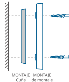
MONTAJE Cuña de montaje de 15°
