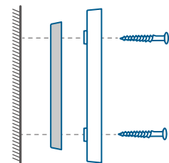
MONTAGE DER MONTAGE DER Winkel halterung
