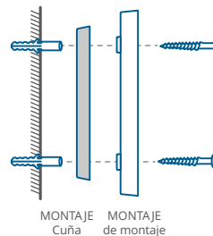
MONTAJE Cuña de montaje de 15°
