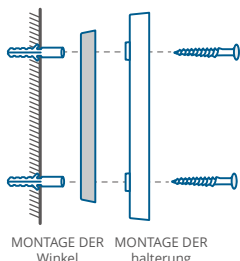
MONTAGE DER Winkel MONTAGE DER halterung Mit 15° Montagewinkel
