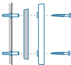
MONTAGE wig MONTAGE beugel
