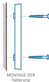
MONTAGE DER halterung Ohne Montagewinkel von 15°
