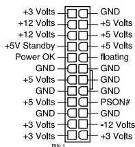
C ATX_PWR
