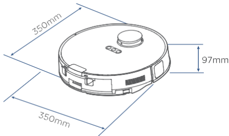
Robot aspirapolvere
