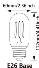
E26 Base
