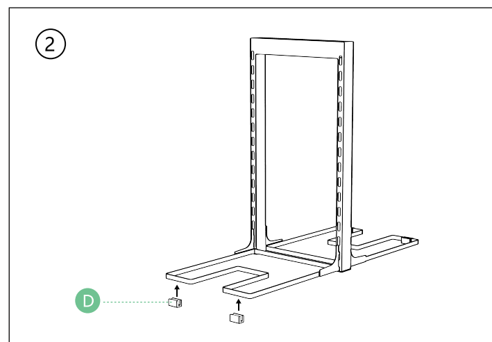
Flip over and install the secure feet (D)
