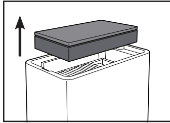
b. Saque el filtro combinado de la unidad. Nota: El prefiltro/filtro de carbón se sujeta al filtro HEPA con una cinta Velcro.
