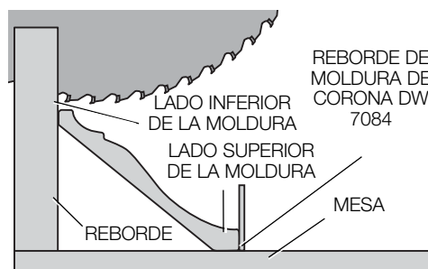
MOLDURA DE CORONA ENTRE REBORDE Y MESA
