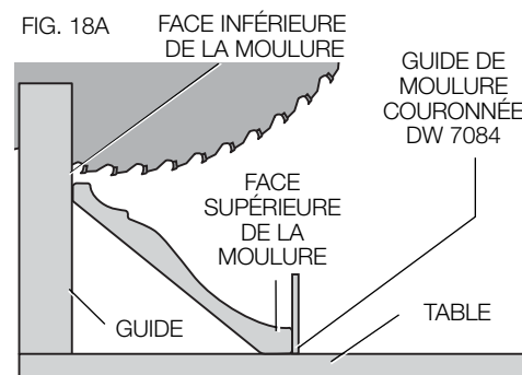
MOULURE COURONNÉE ENTRE GUIDE ET TABLE
