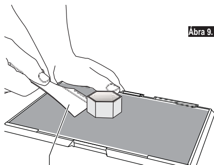
Tárgyleválasztó eszköz
