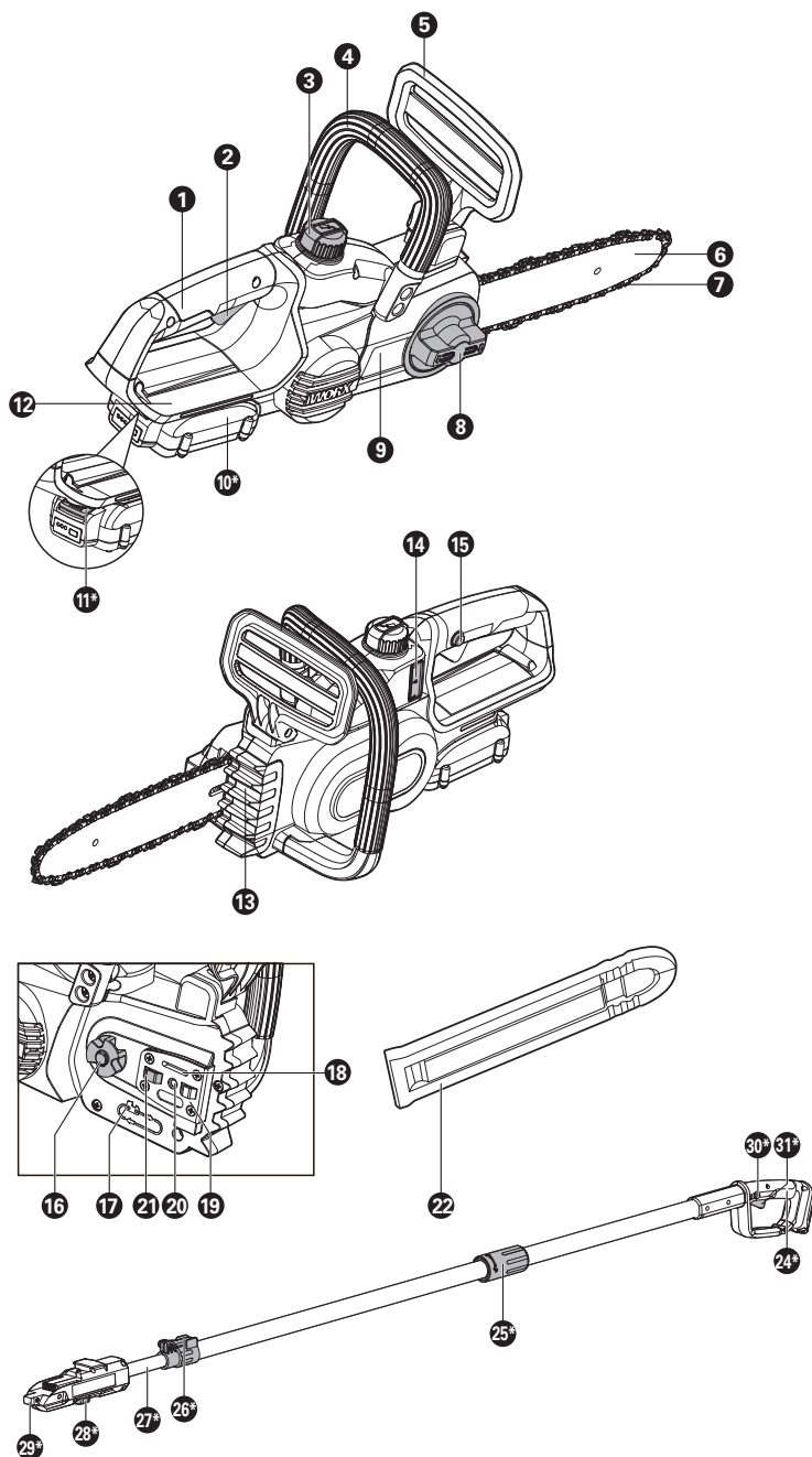
Tronçonneuse sans fil 20 V, Scie d'élagage sur perche 20 V 10 po à batterie (WG322 WG322.X WG323 WG323.X)
