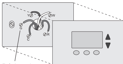
Désignation des bornes
