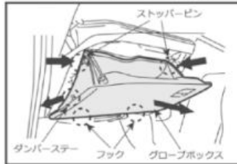
ダンパーステーを取り外し両端から押えてストッパーピンを外し、グローブボックスを引いてフックを外し取り外します。
