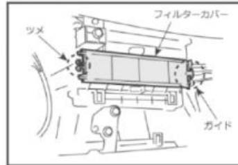
ツメを外しガイドから引き抜き、フィルターカバーを取り外します。
