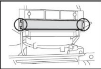
奥にフィルターカバーが見えるので、フィルターカバーのロックノブ（2ヶ所）を解除して、フィルターケースを引き出します。
