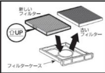
古いフィルターを取り外し交換します。取り付けの際は UP マークが上向きになるように取り付けます。
