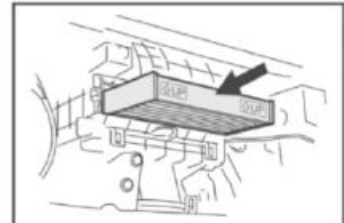
古いフィルターを取り外し、新しいフィルターと交換します。取り付けの際は UP マークが上向きになるように取り付けます。
