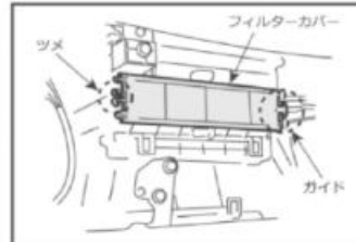
ツメを外しガイドから引き抜き、フィルターカバーを取り外します。
