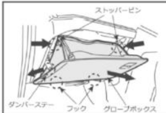
グローブボックスを開き、ダンパーステーを取り外します。両端から押えてストッパーピンを外し、手前に引いてフックを外し全体を取り外します。
