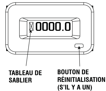
Figure 9 - Horomètre
