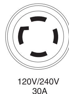
Figura 12 - Receptáculo de 120/240 VAC, 30 Amp
