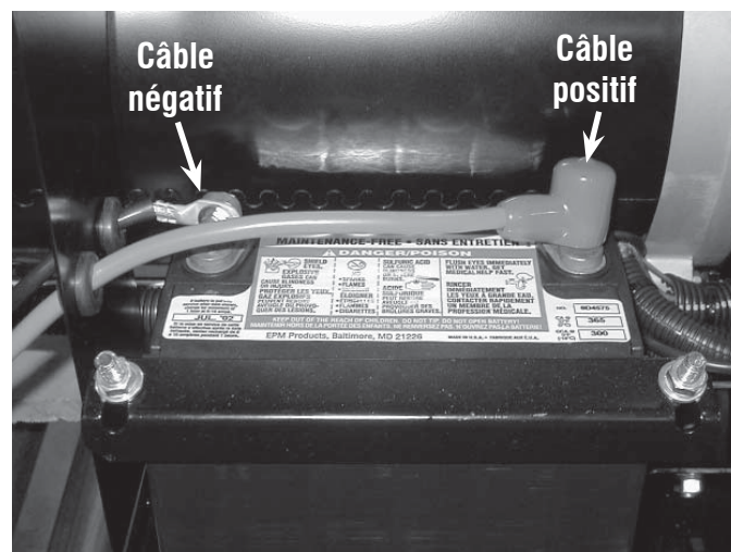
Schéma 3 - Branchements de la batterie
