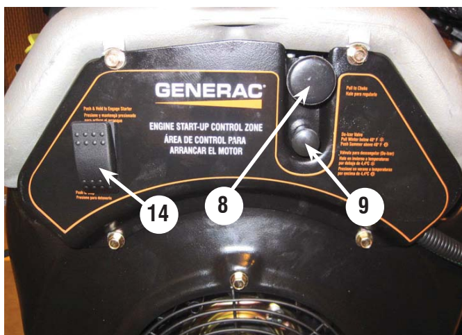
Figura 6 - Panel de control del motor
