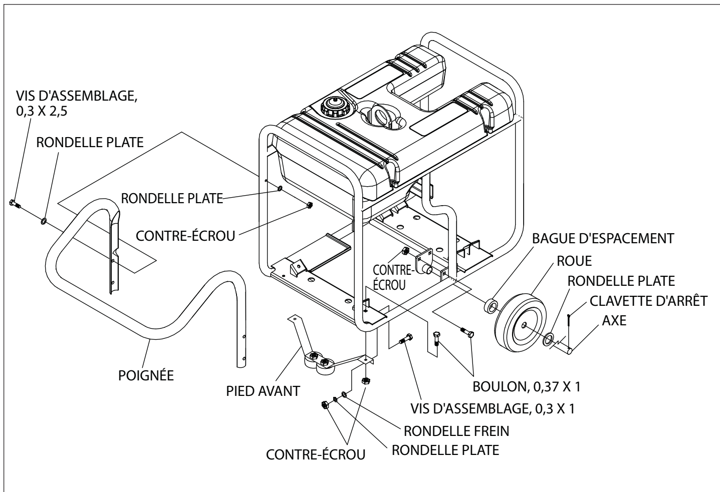
Schéma 2 - Montage de la poignée
