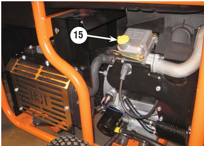
Schéma 7 - Remplissage d'huile
