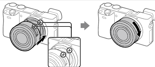
Monteringsmärken
