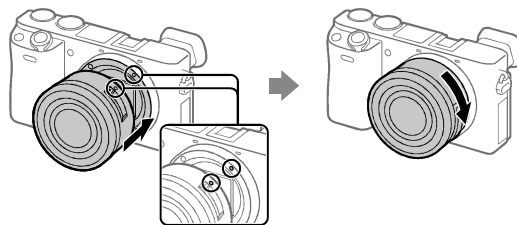
Kiinnitinindeksit
