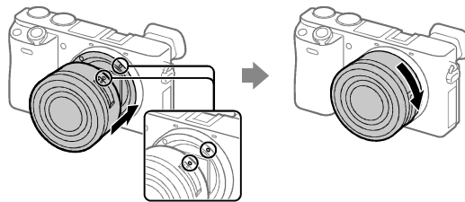
Fatningsindekser
