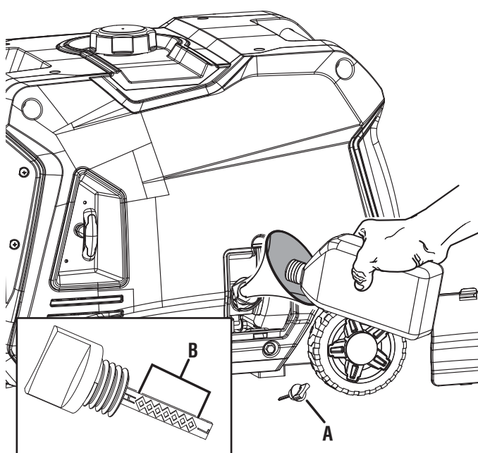
A - Varilla de nivel de aceite
