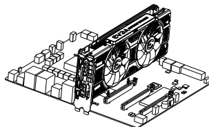
最初の PCI Express x16 スロットへ 2 つ目の GeForce グラフィックカードを差し込んでください。
