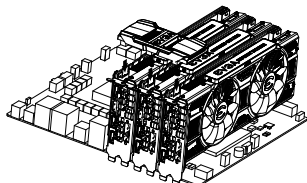
SLI de 3 vias: Instale o terceiro cartão GeForce no terceiro slot PCI Express da placa-mãe. Ligue as placas GeForce usando o conector de ponte SLI 3-way que veio com sua placa-mãe SLI-ready.
