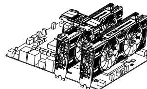
双方向 SLI: 2 つ目の GeForce グラフィックカードを第 2 の PCI Express x16 スロットにインストールします。SLI 対応マザーボードに付属の 2 ウェイ SLI ブリッジコネクタ/新しい 2 ウェイ SLI ブリッジコネクタを使用して 2 つのカードを一緒に接続します。
