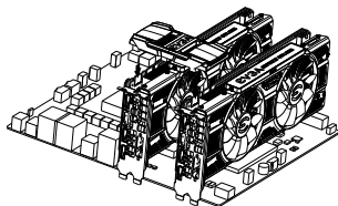
2-way SLI: Instal kartu grafis kedua anda ke dalam slot x16 PCI Express sekunder. Hubungkan dua kartu bersama-sama menggunakan 2-way / 2-way SLI Bridge
