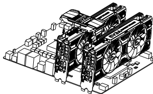
SLI de dos vías: Instale su segunda tarjeta GeForce en la ranura PCI Express x16 secundaria. Conecte las dos tarjetas usando el nuevo puente SLI de 2 vías que viene con su motherboard compatible con SLI.
