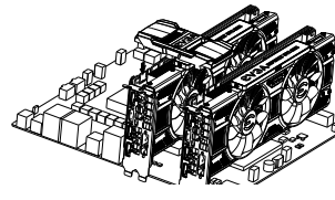
SLI a 2 vie: installa la seconda scheda grafica GeForce nello slot PCI Express x16 secondario. Collega le due schede tra loro utilizzando il connettore bridge SLI a 2 vie fornito con la scheda madre SLI-ready.
