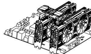
Pont SLI 2-way : Installez votre deuxième carte graphique GeForce dans la fente PCI Express x16 secondaire. Connectez les deux cartes ensemble en utilisant le pont SLI 2-way / le nouveau connecteur Pont SLI compatible avec votre SLI-ready de votre carte mère.
