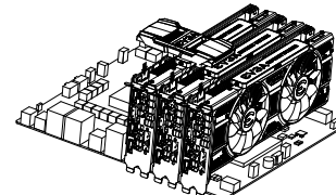
3-way SLI : Installer la troisième carte graphique GeForce dans le PCI Express tertiaire de votre carte mère. Connecter les cartes GeForce ensemble en utilisant le pont connecteur 3-way livré avec votre carte mère SLI-ready.
