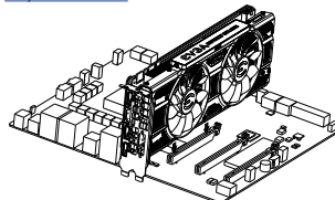
Installa la prima scheda grafica GeForce nello slot PCI Express x16 primario.
