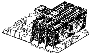
SLI de 3 vías: Instale la tercera tarjeta GeForce en el PCI Express terciaria ranura en la placa madre. Conecte las tarjetas GeForce junto con el conector puente SLI de 3 vías que viene con la placa madre SLI-ready.
