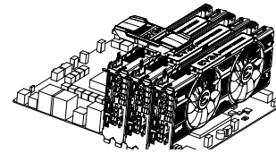
SLI a 3 vie: installa la terza scheda grafica GeForce nello slot PCI Express terziario sulla scheda madre. Collega le schede GeForce tra loro utilizzando il connettore bridge SLI a 3 vie fornito con la scheda madre SLI-ready.
