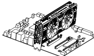
Installer votre première carte graphique GeForce dans le premier port PCI Express x16.
