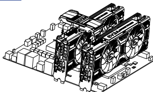
2-way SLI: Instale sua segunda placa de vídeo GeForce no slot PCI Express x16 secundário. Conecte as duas placas utilizando a ponte 2-way SLI/ nova 2-way SLI inclusa em sua placa-mãe compatível com SLI.
