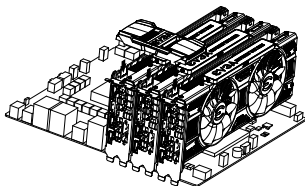
3-way SLI: Pasang kartu grafis ketiga anda ke dalam Slot x16 PCI Express tersier. Hubungkan tiga kartu bersama-sama menggunakan 3-way SLI Bridge.
