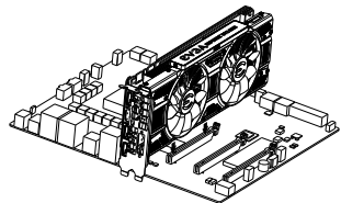
Instale su primera tarjeta gráfica GeForce en la ranura PCI Express x16 principal.
